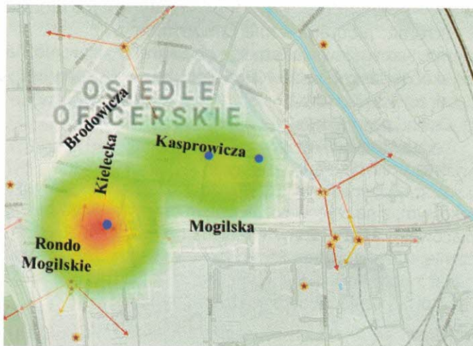
Fragment mapy Grzegórek przedstawiającej wyniki trzech pomiarów natężenia pola elektromagnetycznego
